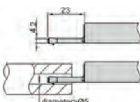
Snímání dotek pro malé otvory ISR-C002-PROBE
