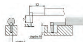
Snímání dotek pro hluboké drážky ISR-C002-DGP
