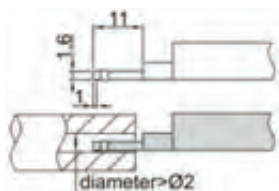
Snímací dotek pro malé otvory ISR-C002-SBP
