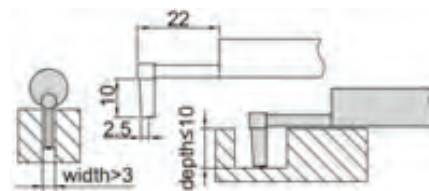
Snímací dotek pro hluboké drážky ISR-C002-DGP
