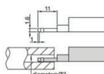
Snímání dotek pro malé otvory ISR-C002-SBP
