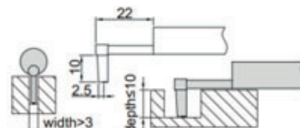
Snímání dotek pro hluboké drážky ISR-C002-DGP
