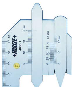
INSIZE 4838-1 svárová měrka.
