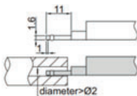
Snímání dotek pro malé otvory ISR-C002-SBP
