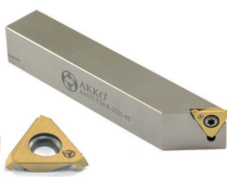
Držáky a přesně broušené destičky pro rohové řemenic
