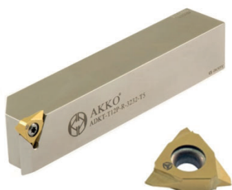
Držáky a přesně broušené destičky pro zapichování řemenic
