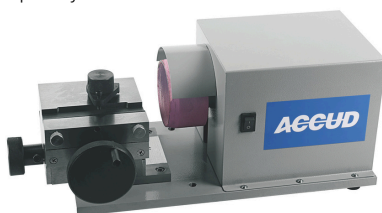
Přístroj pro renovaci dosedací plochy hloubkoměru posuvných měřidel
