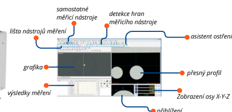
Softwarové rozhraní
