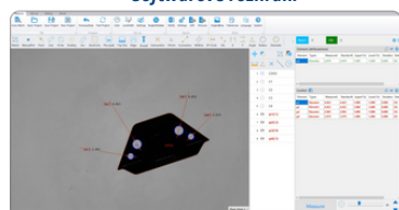
Softwarové rozhraní
