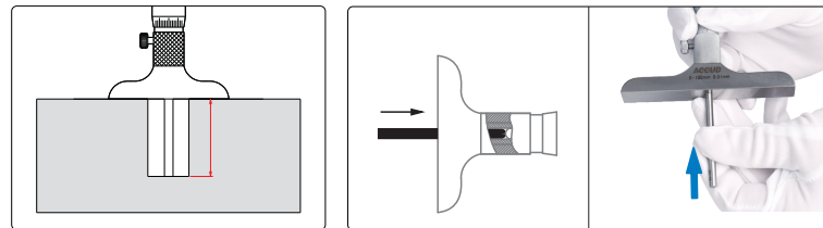
Install rod
